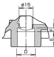
DETAIL "B" (CONDUIT CONN.)
